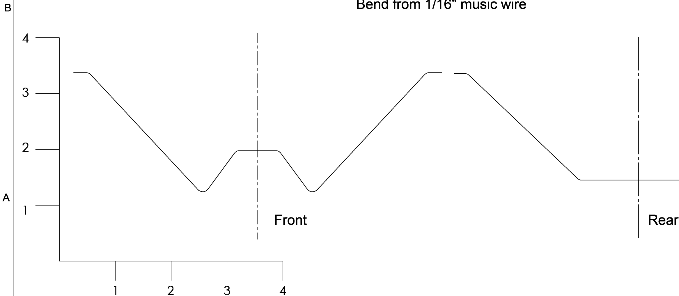
Cabane Strut Bend Templates
